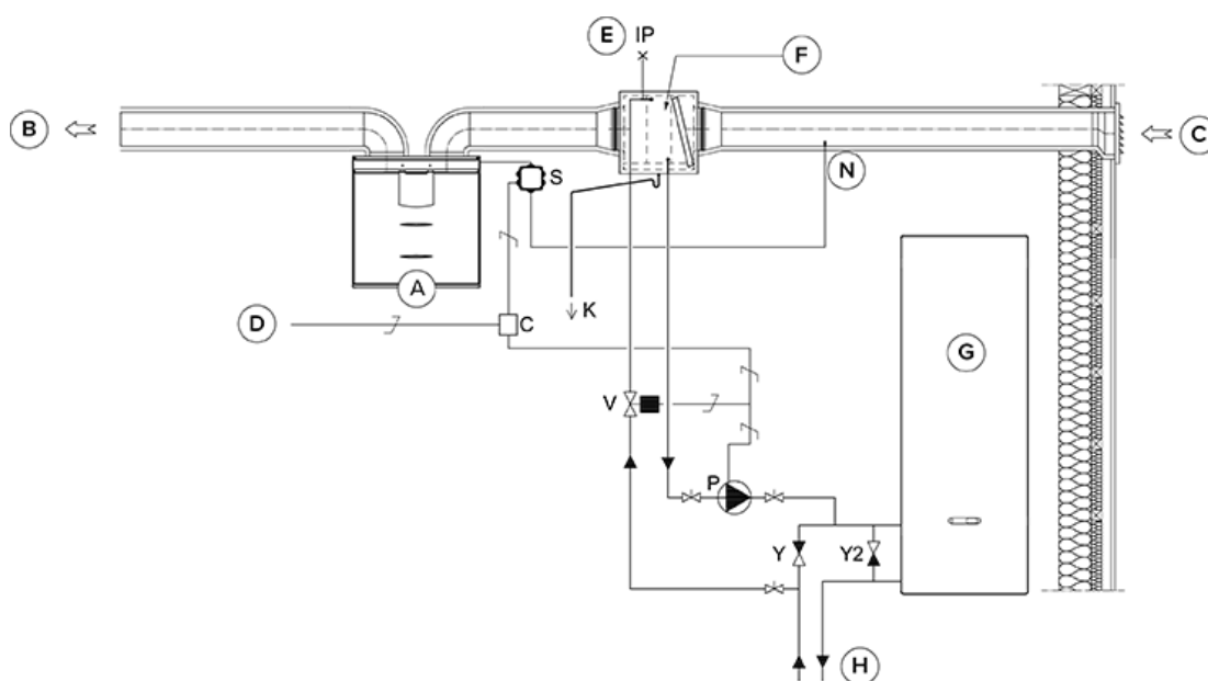
Joonis 6. Kanaliradiaatori talitluskem sissepuhkeõhu kanalis
