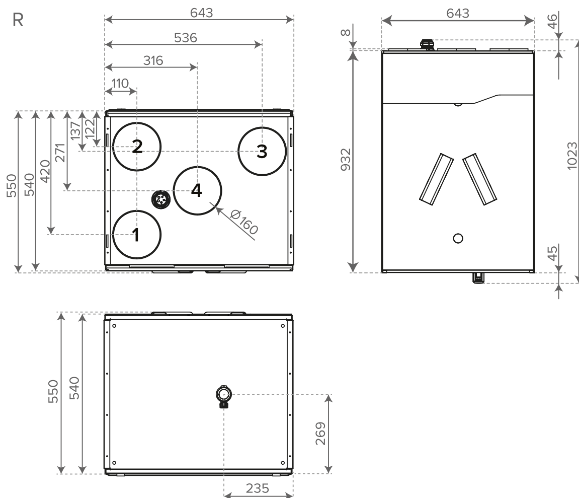
Joonis 8. Mõõtmed ja kanali väljalaskeavad MyVallox 149 CFi L
